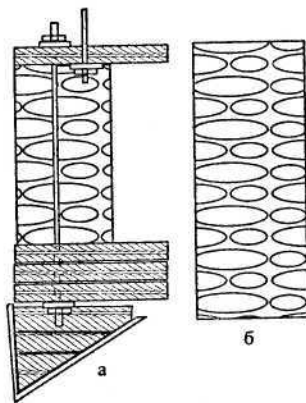
Рис. 5. Разрез стенки каменного колодца: а — промежуточные кольца с анкерами; б — перевязка камней между собой
